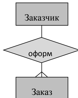
Рисунок 1 – Связь между сущностями Заказчик и Заказ
