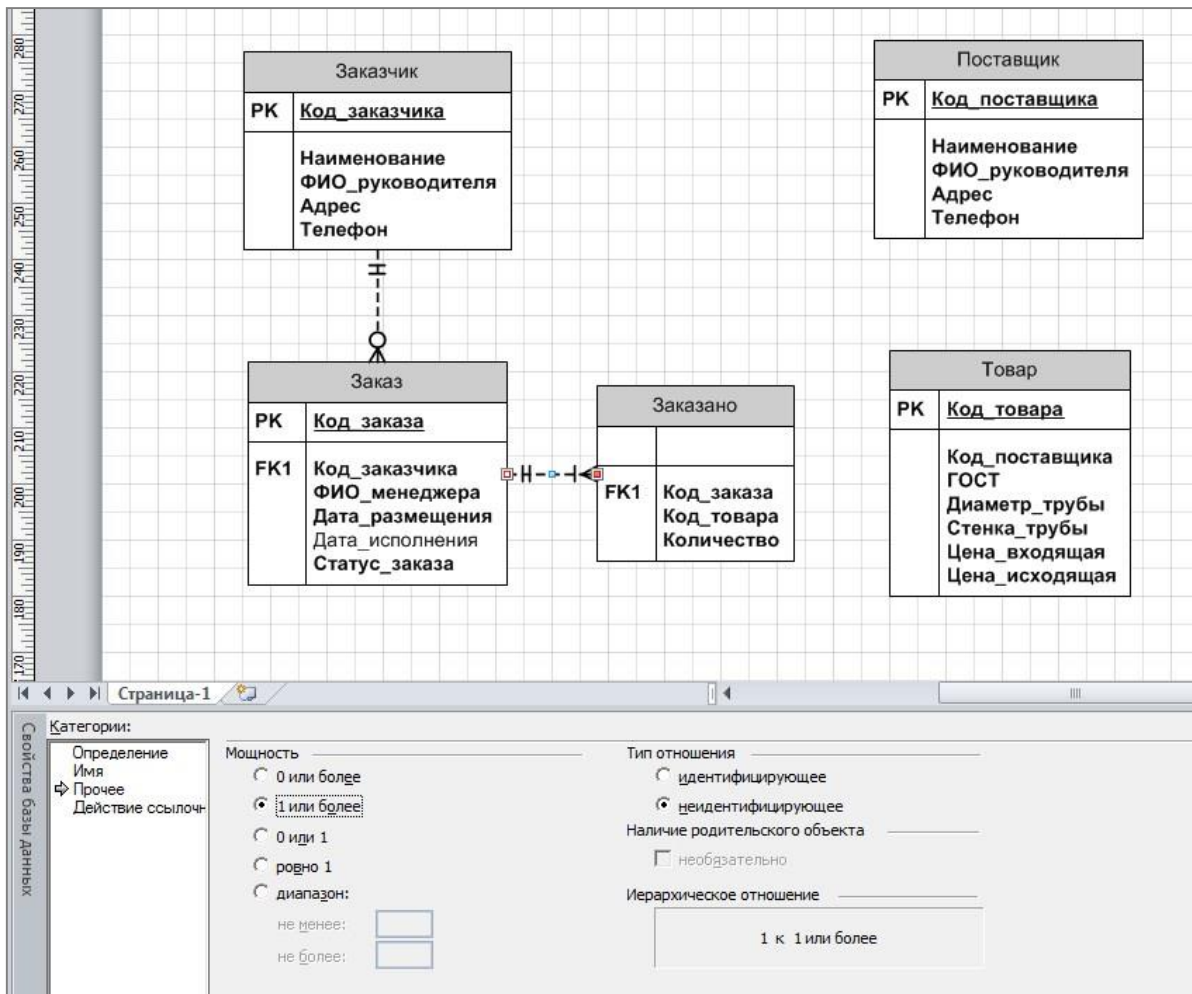
Рисунок 11 – Изменение кардинальности связи.
